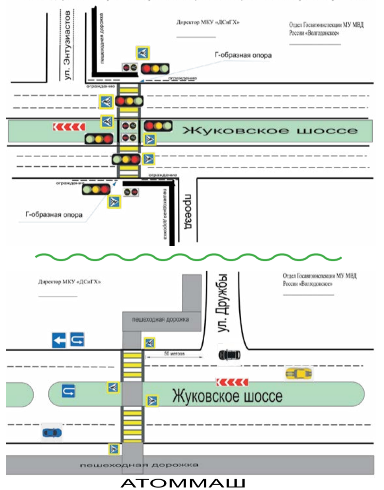
Схема установки светофорного объекта и обустройство пешеходного перехода на автодороге по Жуковскому шоссе в районе пересечения с ул. Энтузиастов
